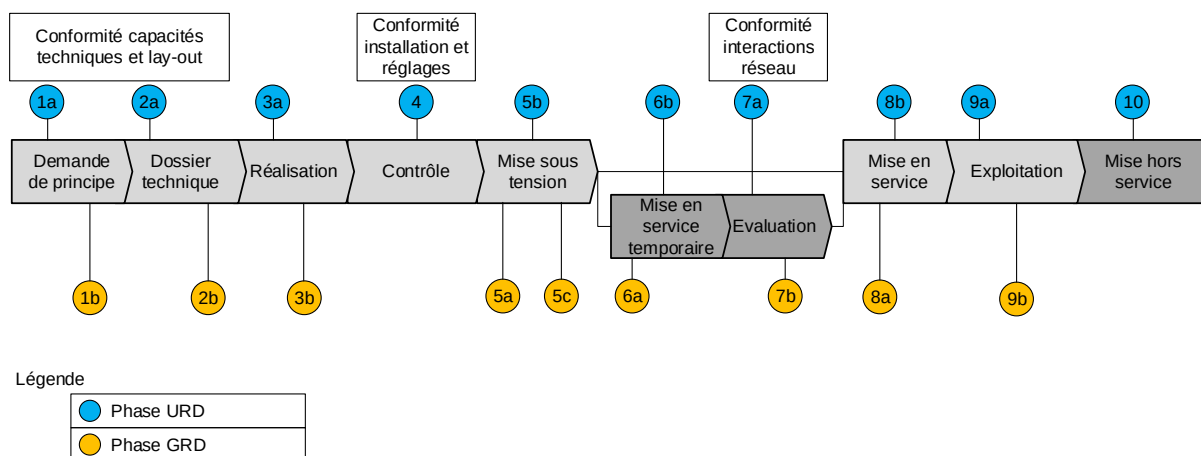
Figure 3 - Procédure standard de mise en service d'une installation de production d'électricité
