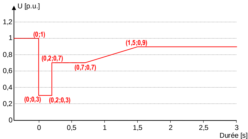
Figure 11 - Profil tension fonction du temps pour une technologie de production d'électricité synchrone
